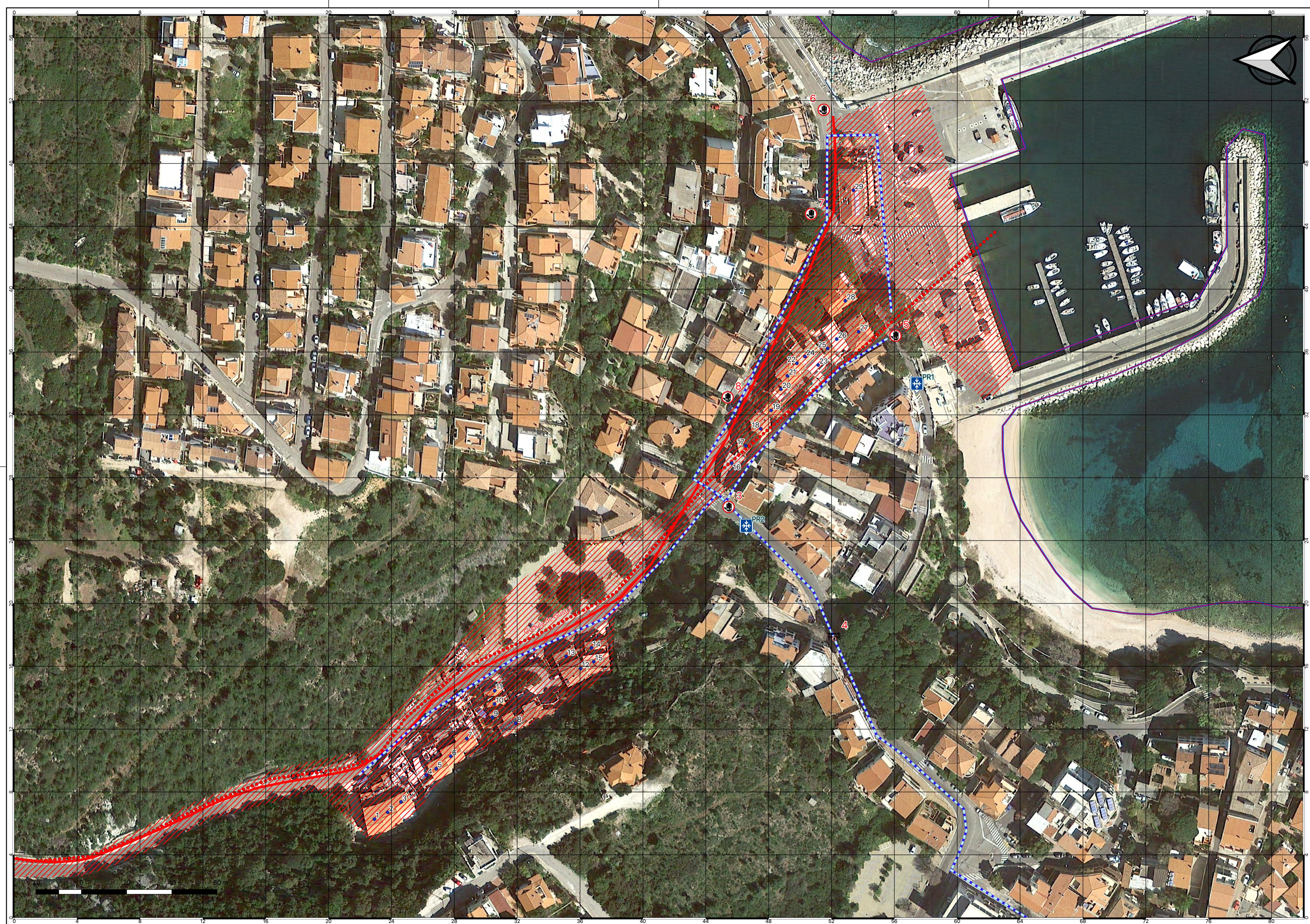
TAV IDRO1 CALA GONONE 2 Rischio IDROGEOLOGICO SCENARIO 1.2 IDROLOGICO su base Google Satellite
